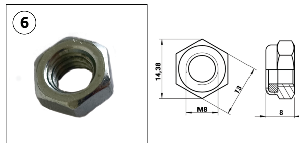
PORCA M8
